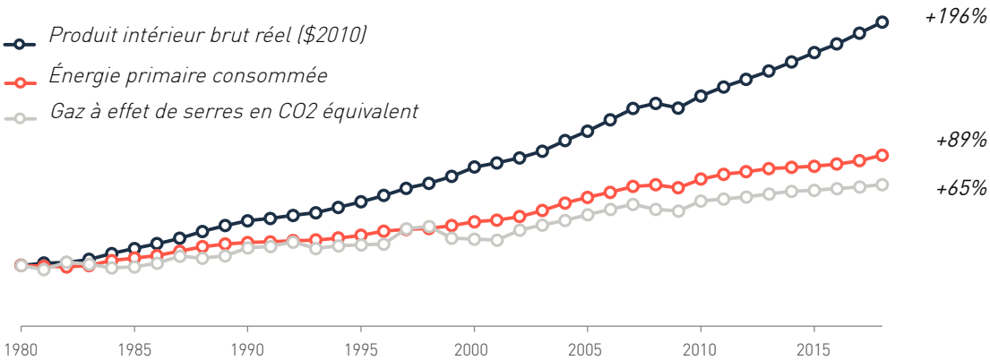
Évolution de la consommation d'énergie primaire, des gaz à effet de serre et du PIB l'échelle mondiale | 1980 - 2018 (base 100 en 1980) - Carbone 4 2
